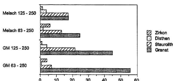
Abb. 2. Schwermineralverteilung in Abhängigkeit von Fraktion und Lithofazies (Kornprozentanteil am Gesamtspektrum). a) Rezent und pleisto-zäne Sedimente (125–250 µm) verschiedener Faziesbereiche (linkes Bild), b) Vergleich verschiedener Fraktionen von rezenten fluviatilen (Melach) und pleistozänen glazialen (GM ... Grundmoräne) Sedimenten desselben Liefergebietes (unteres Bild).
