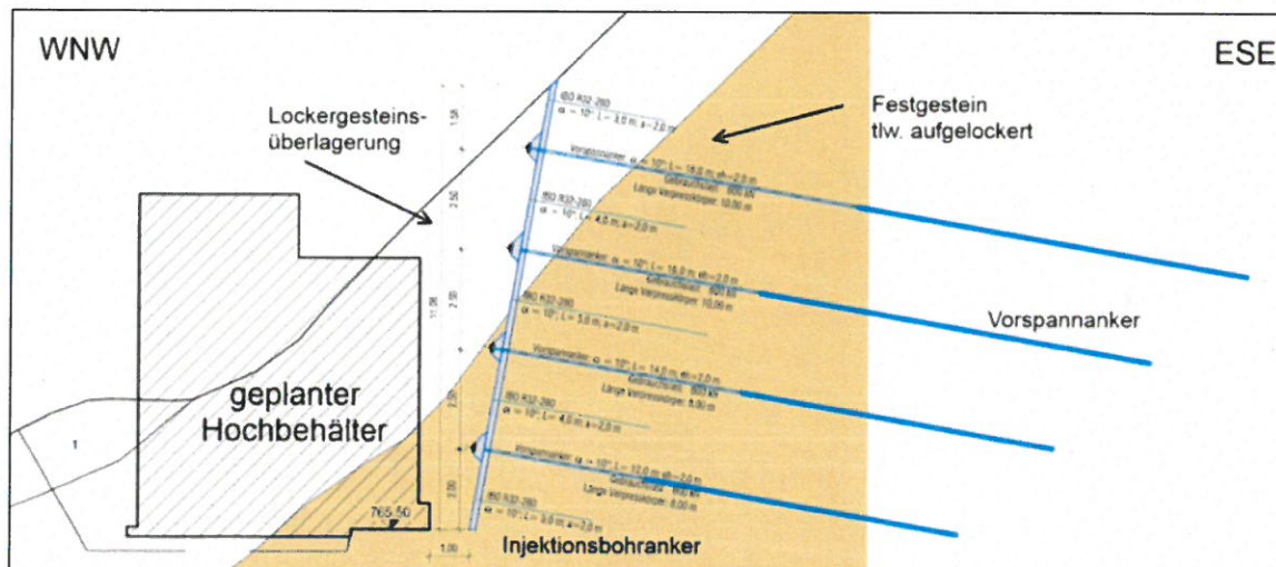
Abbildung 44: geplanter Hochbehälter mit Baugrubensicherung (Ausschreibungsprojekt)
