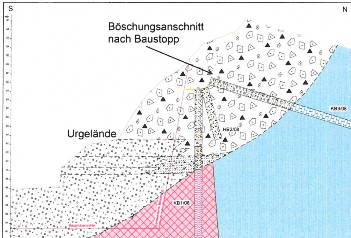
Abbildung 41: Geologisches Profil mit Erkundung und Böschungsanschnitt
