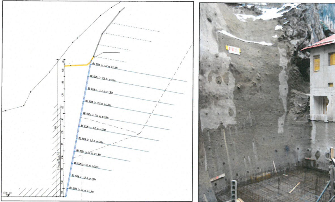
Abbildung 42: Umgeplante und ausgeführte Nagelwand bergseitig des Krafthaus
