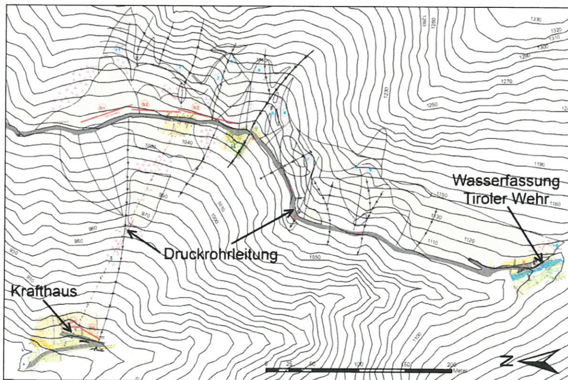
Abbildung 39: Detailkartierung Naturgefahren
