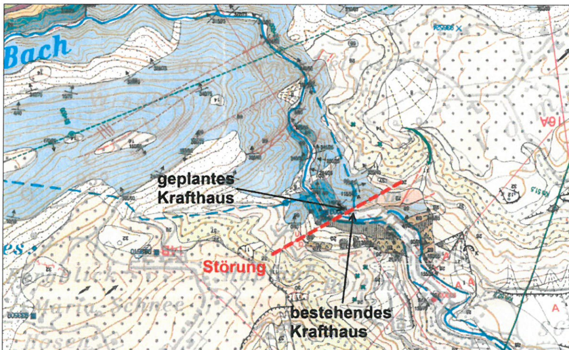
Abbildung 40: Bestehende geologische Karte im Projektraum (BEG)
